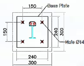
T. ATAS BASEPLATE
