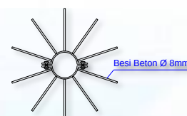
ANTI PANJAT
